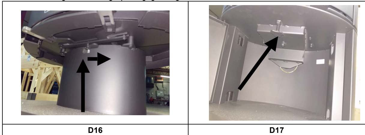
Abbildung 3: Sicherungssperre gegen ungewolltes verdrehen des Kaminofens
